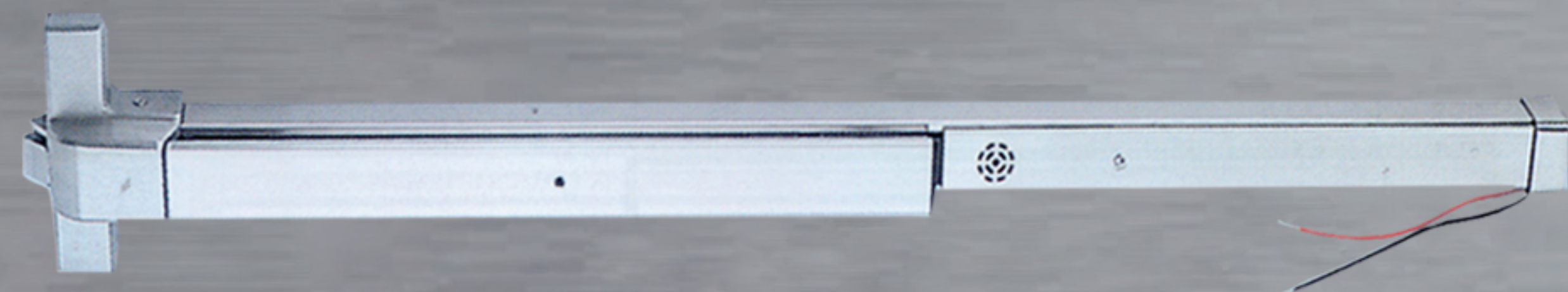
Panic Exit Device Rim Type(Alarm Function) คานผลักแบบธรรมดา ผิวสแตนเลส มีสัญญาณเตือน TYPE : PR2P
